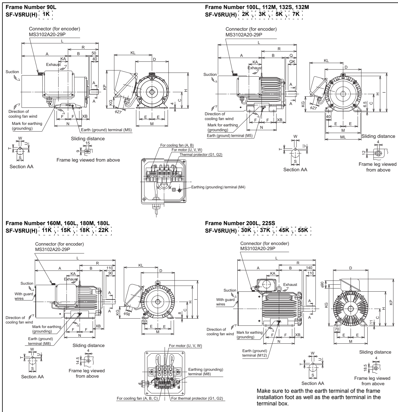
Dimensions table
