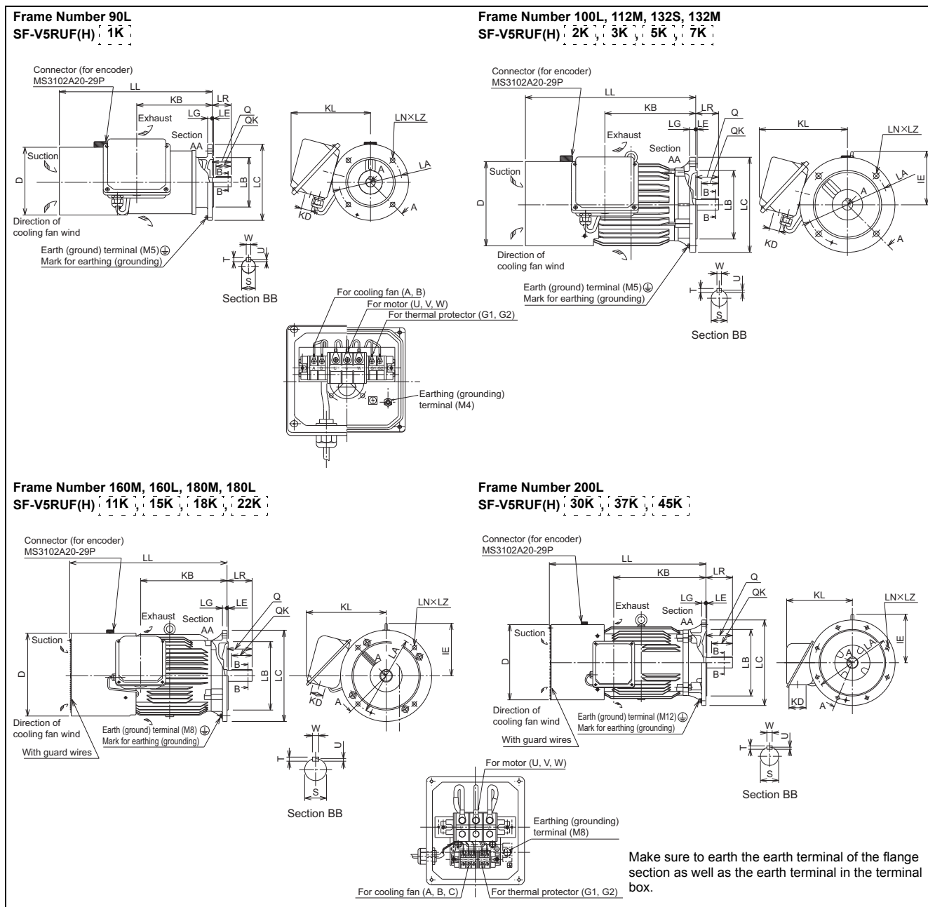
Dimensions table
